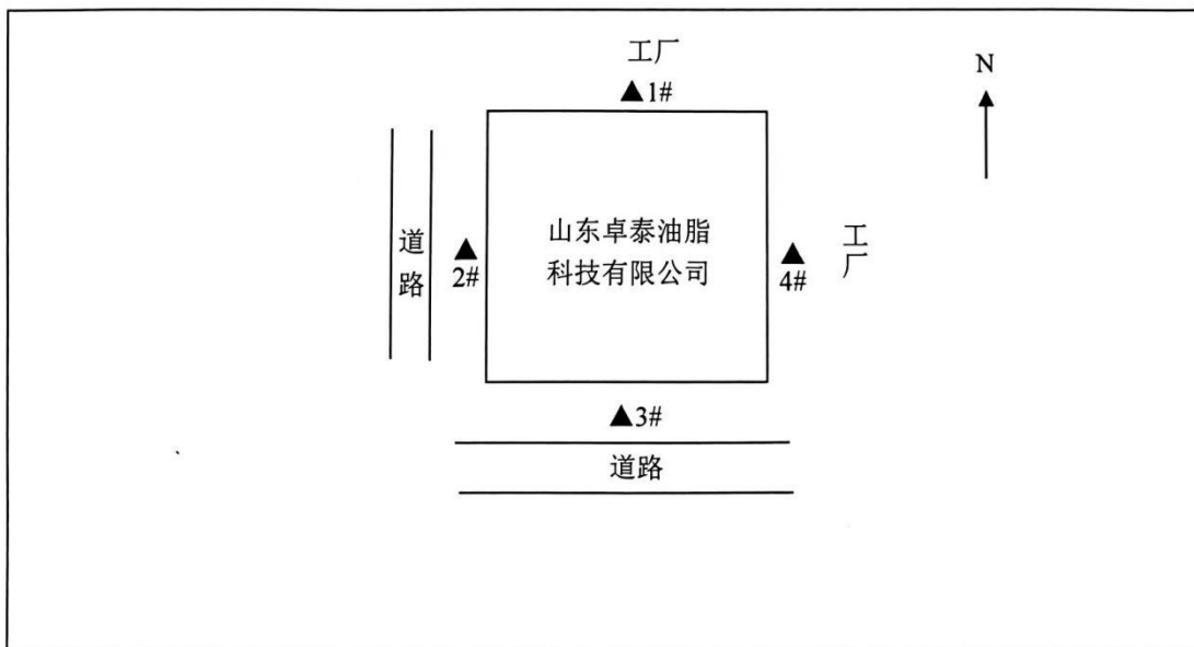
附图：厂界外 1m 噪声测点示意图
